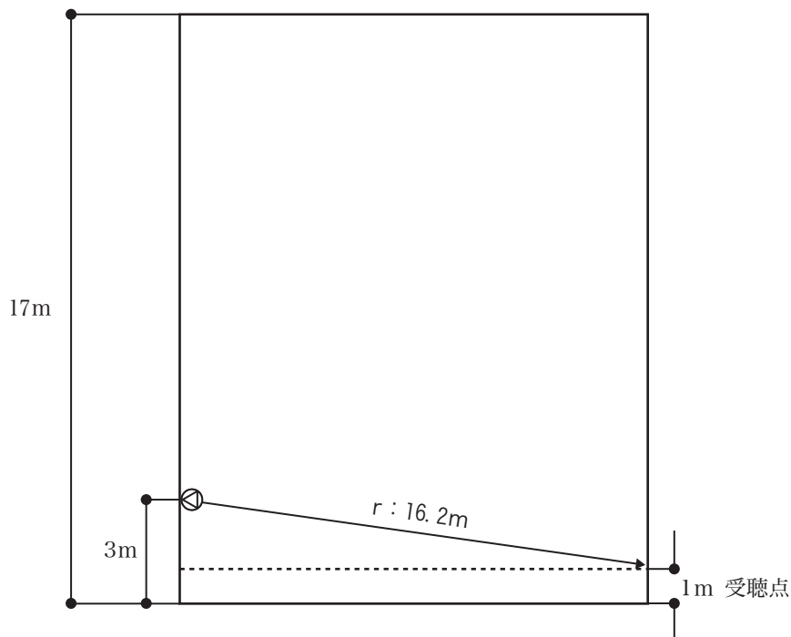
〔側面図〕
